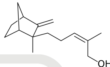
\beta -santalol
