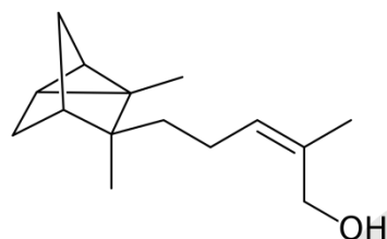
\alpha -santalols
